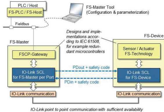
Fig. 8: SCL layer stacks
